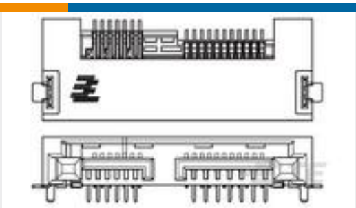
TE 零件编号2129115-3 SLIMLINE SATA PLUS PLUG AU G/F
