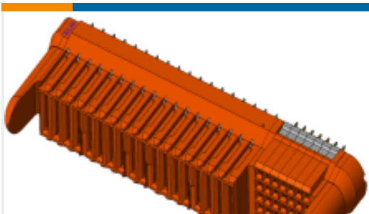
TE 零件编号1-1892787-0 Assy Vert MINIPAK HDL Rcpt 35s18p
