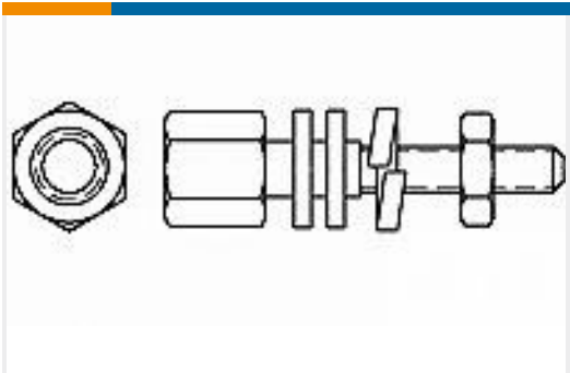
TE 系列/零件编号5747223-3 AMPLI FEM S'LOCK KIT
