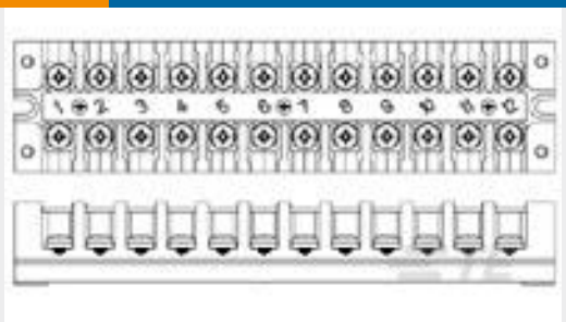
TE 系列/零件编号3- 1437381-5 2B112N=1 PIECE TERMINAL BLOCK
