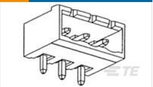
TE 系列/零件编号796639-7 7POS 5.08MM CE R/A HDR,TRM BLK
