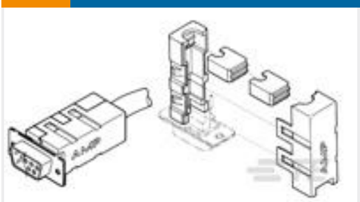
TE 系列/零件编号3-747579-4 SHLDNG FERRULE, PLTD, BULK PKG
