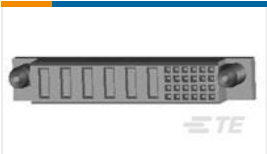
TE 系列/零件编号6450541-4 MBXL VERT RCPT 24S+6P
