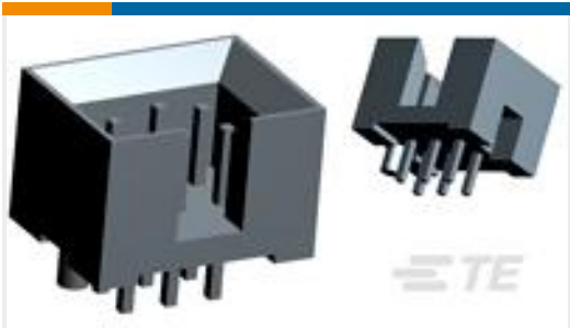
TE 系列/零件编号2041540-1 2.0mm Box Header, 6 Pos. Vertical, DIP
