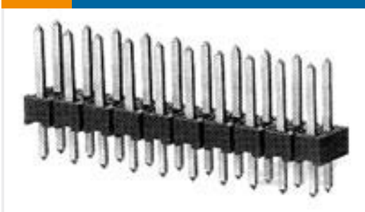
TE 系列/零件编号103777-2 04 MODII HDR DRST B/A .100CL
