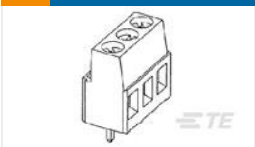
TE 系列/零件编号1-282841-7 TERM-BLOK PCB W. LOCK 5.08 mm
