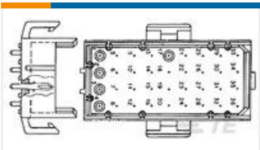
TE 系列/零件编号1-608017-4 36 POS MR HEADER ASSY SPCL LF
